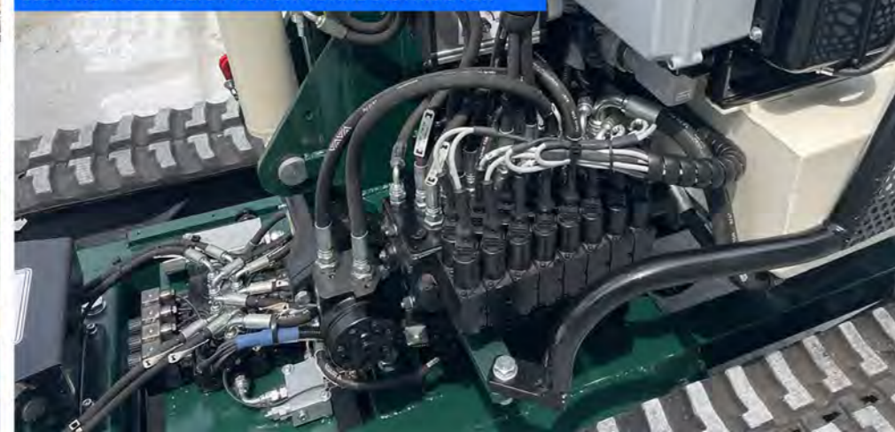
DISTRIBUTORE ELETTRO-IDRAULICO PROPORZIONALE ELETTRO-HYDRAULIC PROPORTIONAL DISTRIBUTOR
